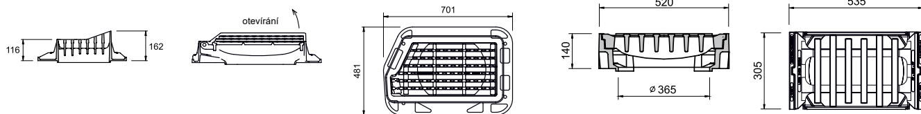
mříž + rám KM11RD pro přímé zabudování do Curb Kingu
