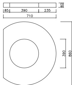
vyrovnávací prsteneč TBV-Q 390/60
