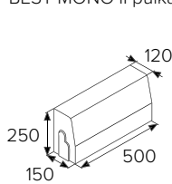
BEST MONO II půlka
