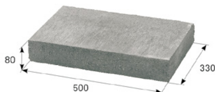
BEST PŘÍLOŽNÁ DESKA
